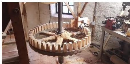
1e kamwiel onderaandrijving maalstoel
